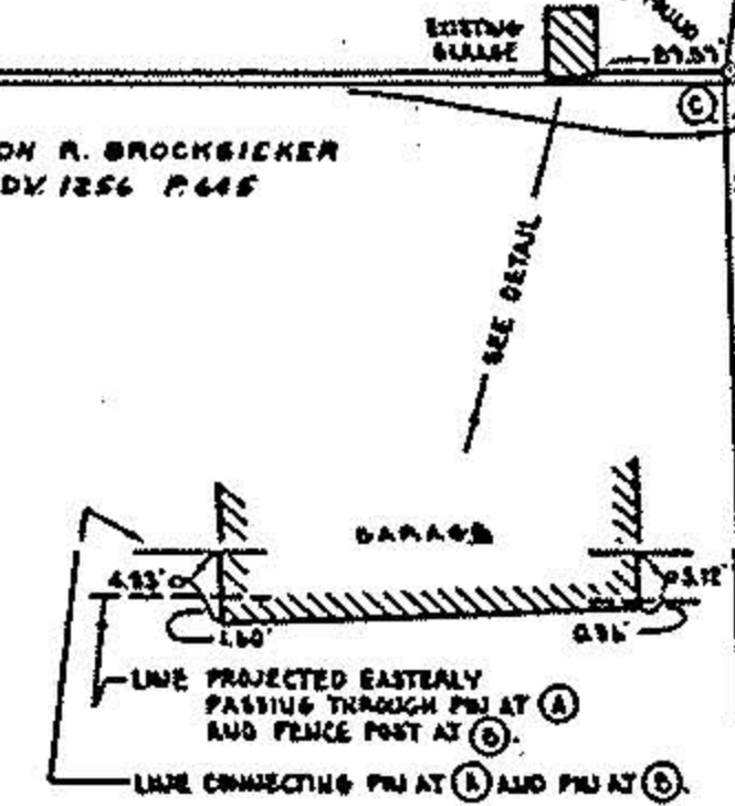
DETAIL SCALE: 1" = 10'
